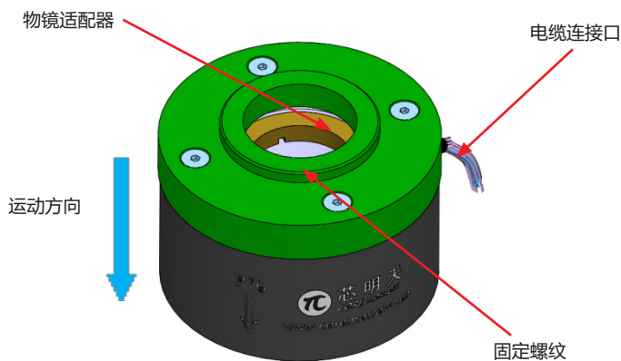
图 1 P76 压电物镜定位器组成和运动方向
