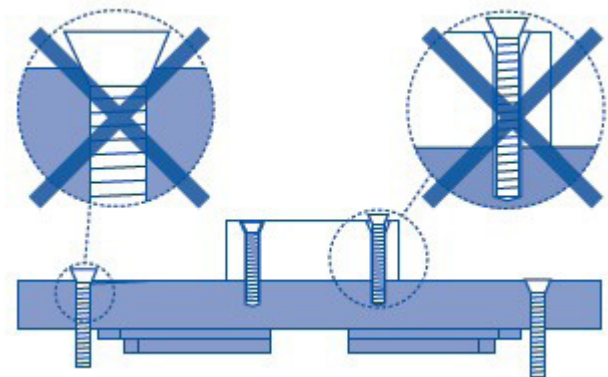
图 9 不恰当的螺栓选择
