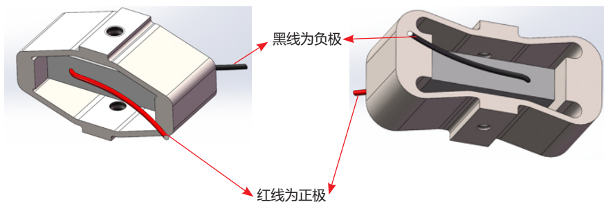
图 2 连接示意图
