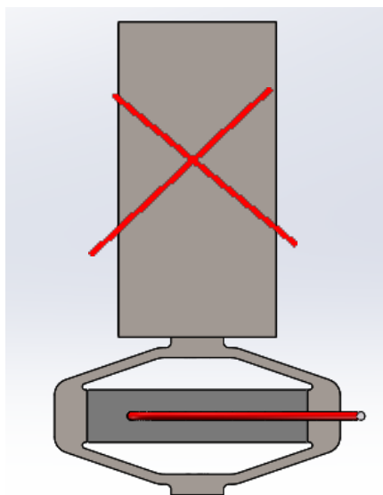
图 6 尽量不要让负载重心远远超过运动面
