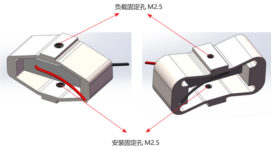
图 3 安装示意图
