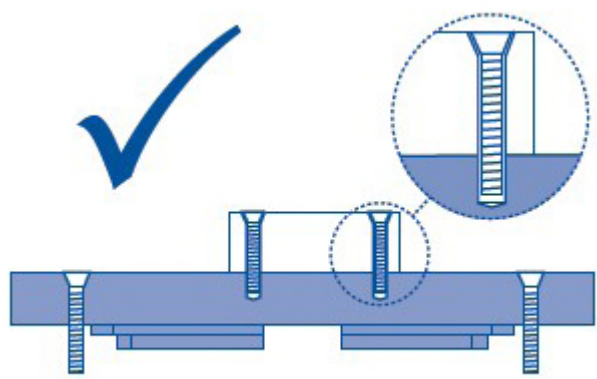
图 8 正确的螺栓连接方式
