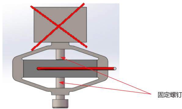
图 7 固定螺钉过长损坏压电陶瓷
