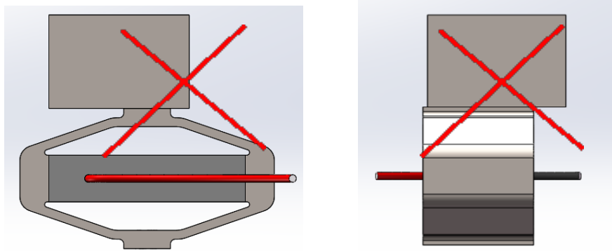
图 5 禁止加载负载在放大机构的一侧
