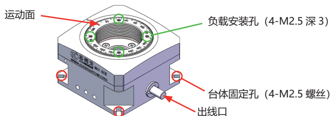
图 1 N61.R5E 压电旋转平台
