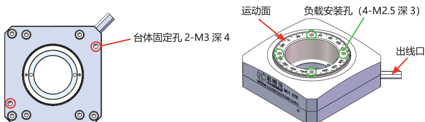
图 2 N61.R5K 压电旋转平台
