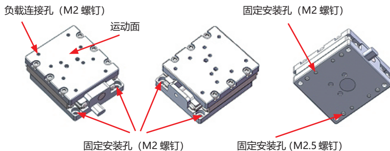
图 2 安装示意图
