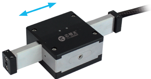
图 1 N31 压电马达运动方向
