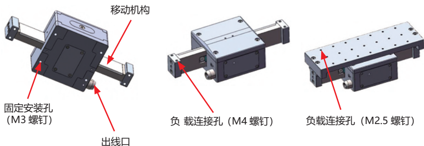
图 2 N31 安装示意图
