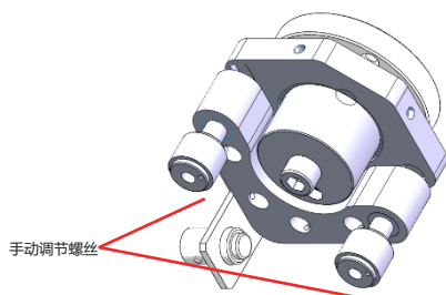
图 2 手动调节转角
