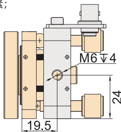
图 3 安装螺钉示意图
